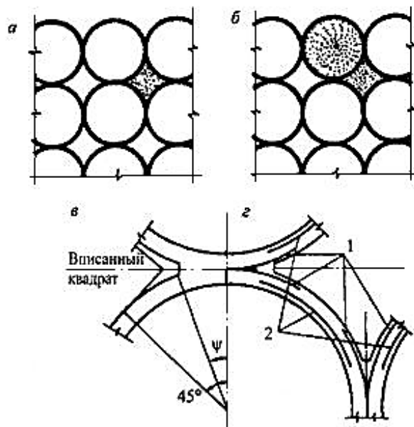
Рисунок 8 - К расчету звездочки
