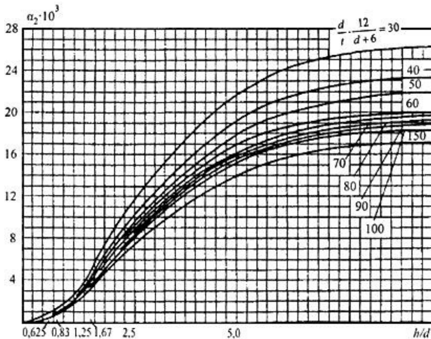
Рисунок 7 - Значения коэффициента, учитывающего влияние локальных давлений сыпучих материалов, моментов, рассчитанных по формулам (11) и (17)
