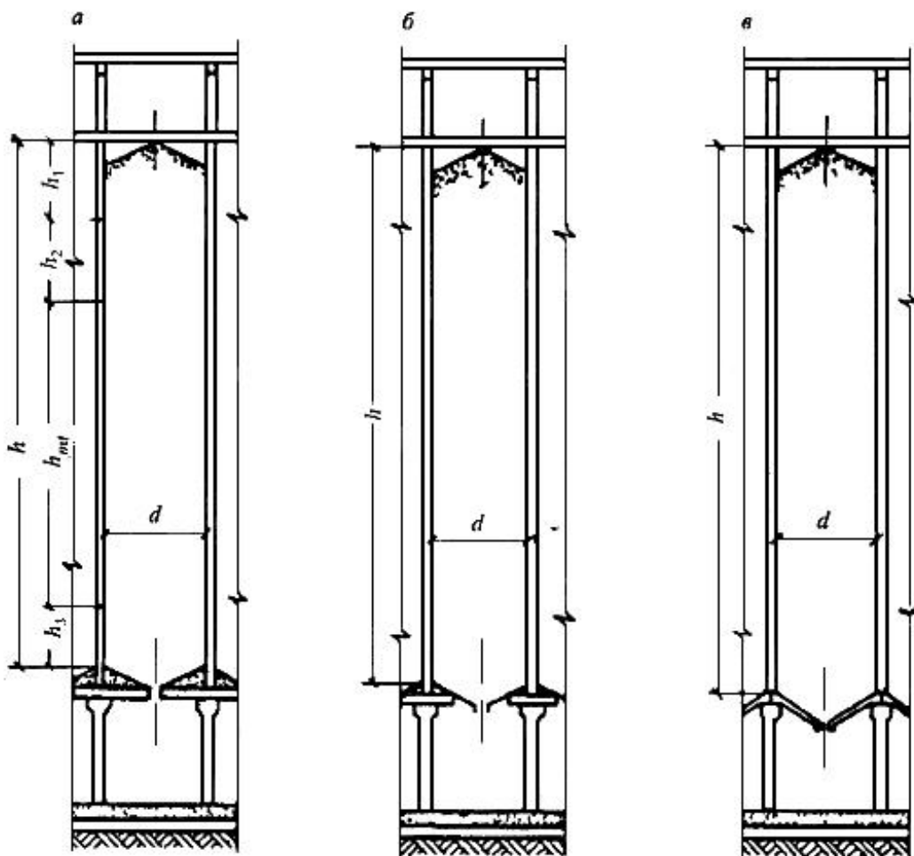
Рисунок 1 - Разрезы силосов
