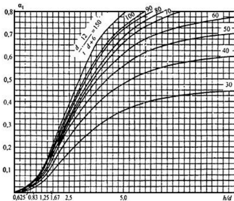
Рисунок 7 - Значения коэффициента, учитывающего влияние локальных давлений сыпучих материалов, моментов, рассчитанных по формулам (11) и (17)
