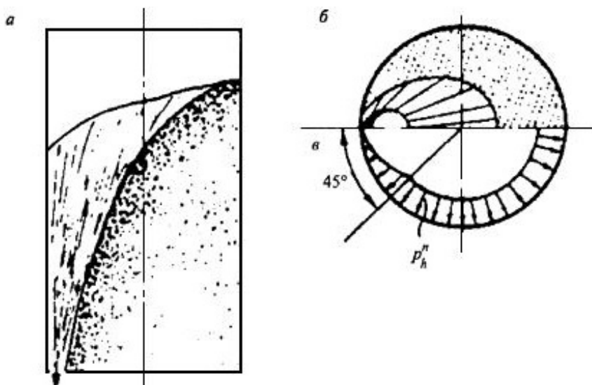
Рисунок 5 - Схема распределения горизонтального давления
