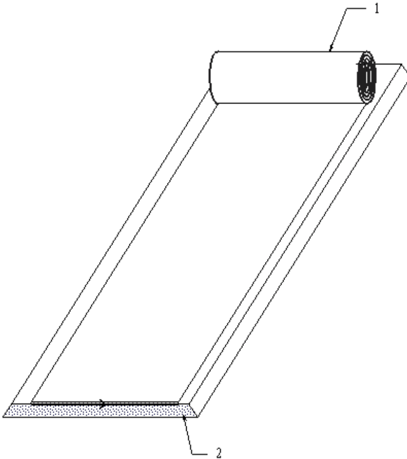
Рис. 2. Устройство горизонтальной гидроизоляции: 1 – укладываемая гидроизоляция; 2 – подбетонка
